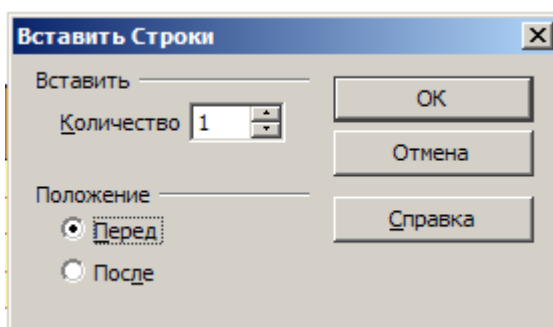
Рисунок 20. Вставка строки
