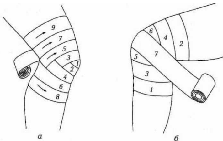
Рисунок 5. «Черепашня» повязка
