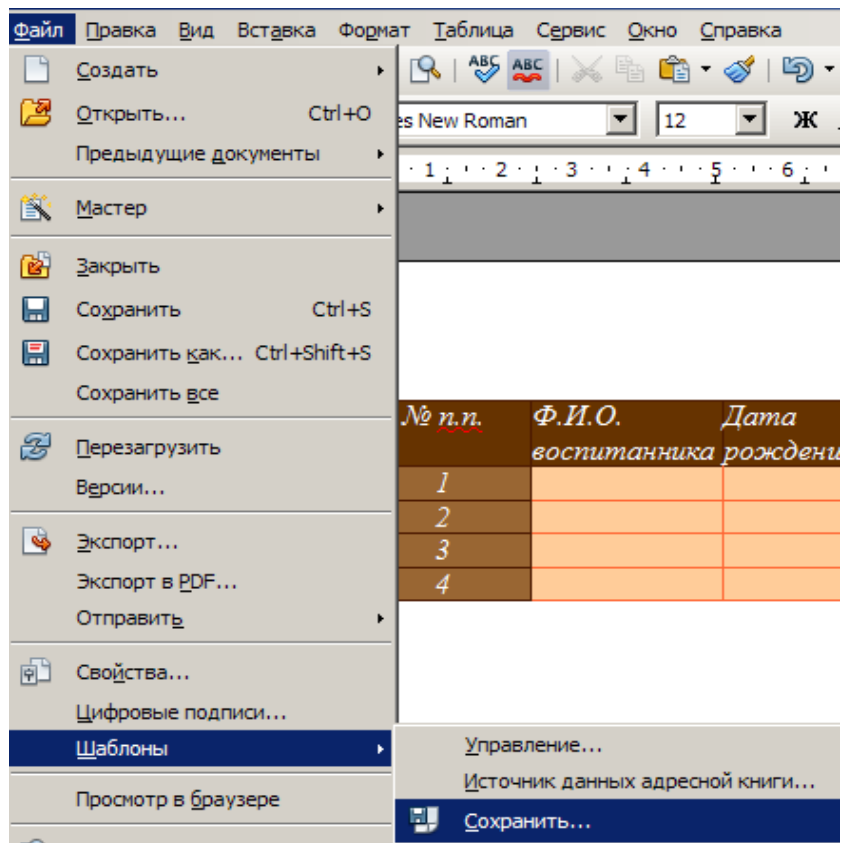
Рисунок 4. Таблица задания 1
