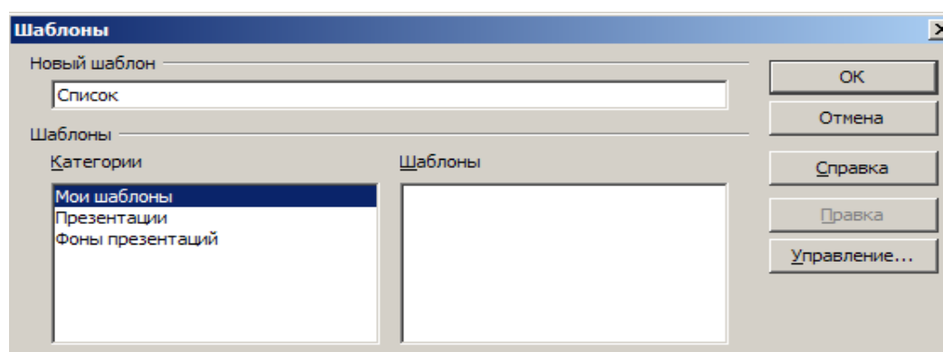
Рисунок 6. Окно Шаблон
