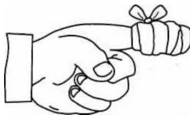
Рисунок 3. Спиральная повязка
