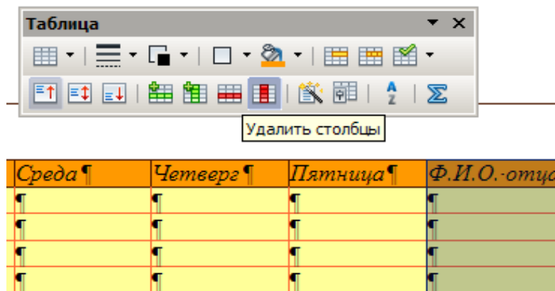
Рисунок 19. Удаление столбца
